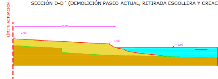
SECCIÓN D-D' (DEMOLICIÓN PASEO ACTUAL, RETIRADA ESCOLLERA Y CREACIÓN DE PLAYA NUEVA)
