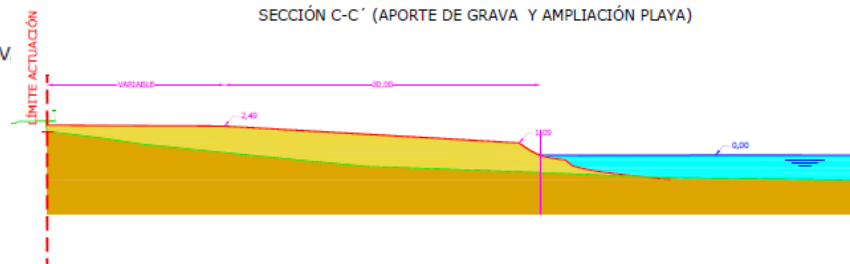
SECCIÓN C-C' (APORTE DE GRAVA Y AMPLIACIÓN PLAYA)
