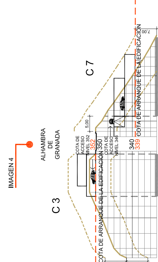
SECCION 20
